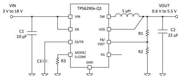
簡略回路図
