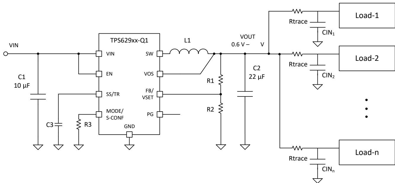
図 9-65. Multiple Loads
