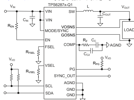
概略回路図
