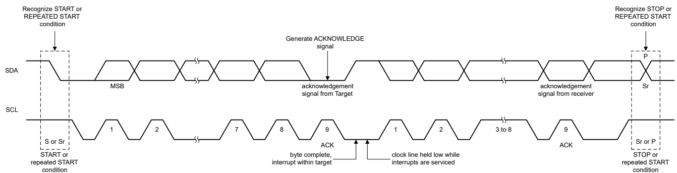
図 8-20. Bus Protocol
