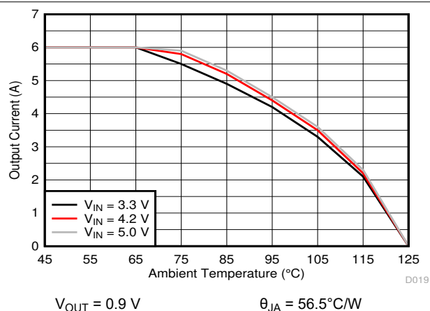
9-10. Thermal Derating
