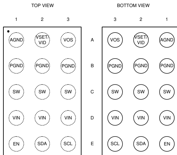
図 6-1. YCG (15 Pin)
