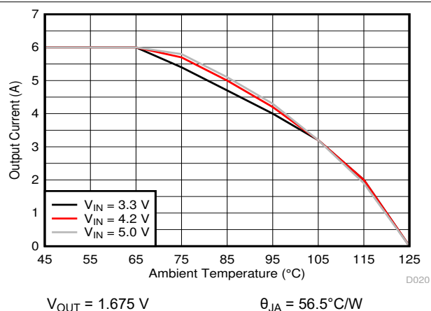
9-11. Thermal Derating
