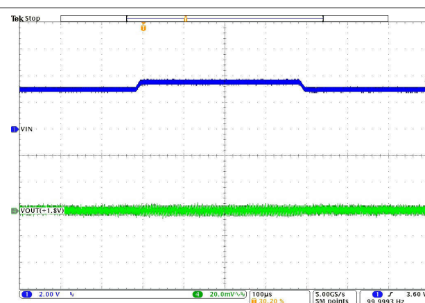
図 8-36. Line Transient
