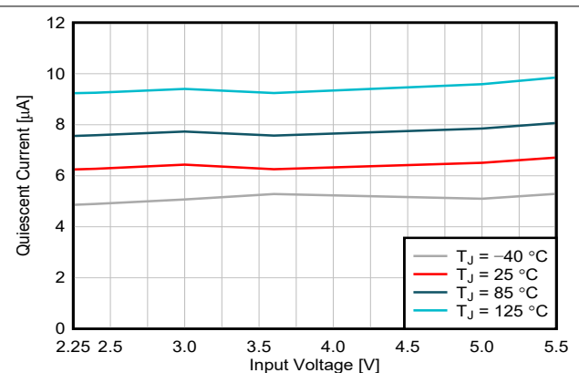
図 6-4. Quiescent Current
