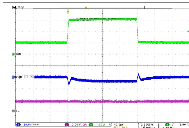
図 8-33. Load Transient
