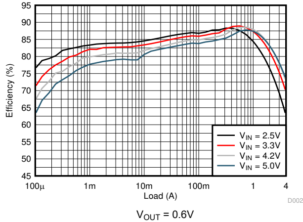
図 8-3. Efficiency
