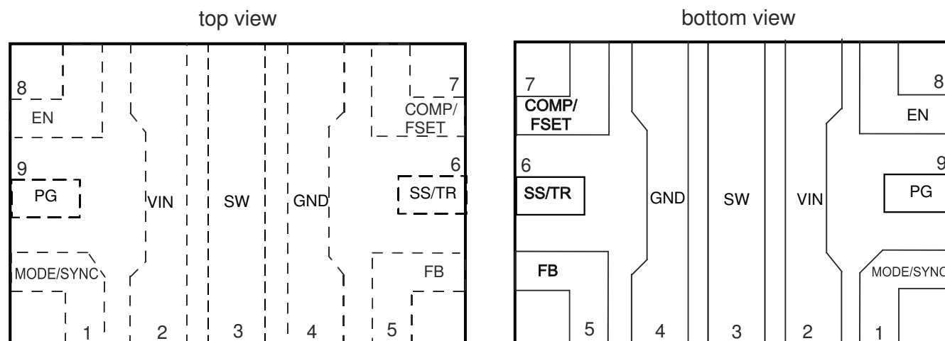
図 5-1. RWY パッケージ、9 ピン (VQFN)
