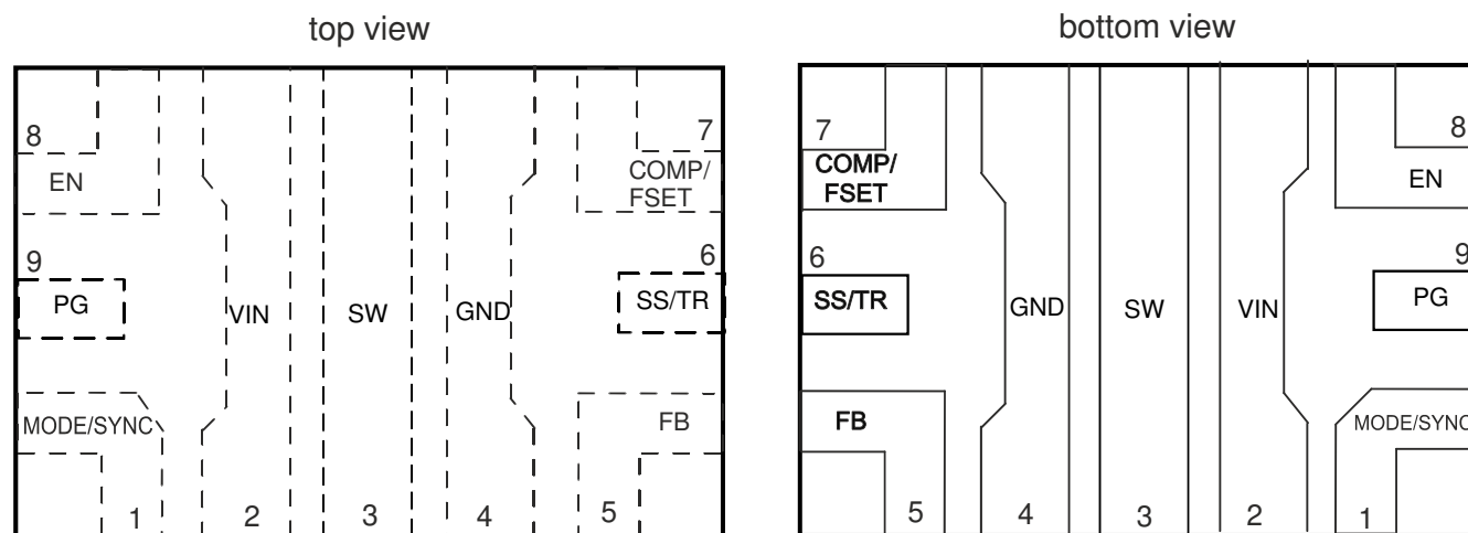
図 6-1. RWY Package 9 Pin (VQFN)
