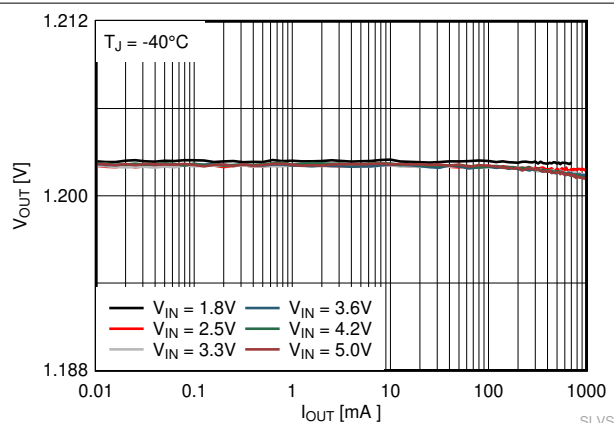
TPS62801 起動後、VSEL/MODE = High V OUT = 1.2 V 強制 PWM モード T J = -40°C
