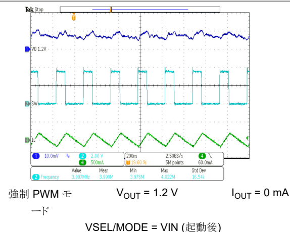
図 8-30. TPS62801 代表的な動作、強制 PWM モード
