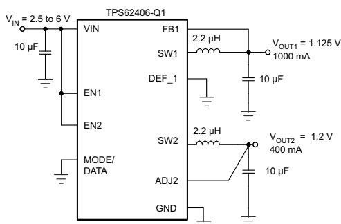
概略回路図
