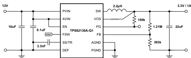
代表的なアプリケーションの回路図
