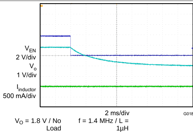
图 24. Shutdown
