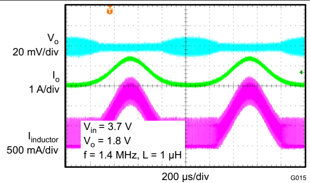
图 19. PFM Operation
