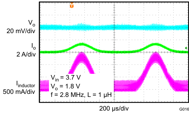
图 22. Load Sweep
