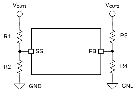
図 7. Output Voltage Tracking
