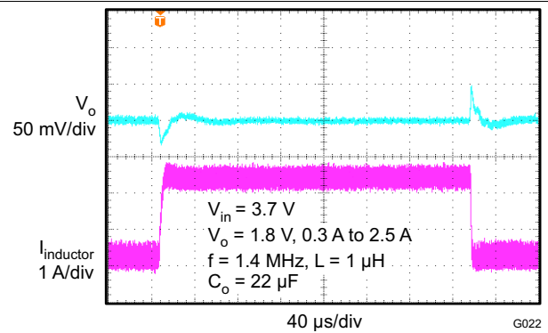
图 27. Load Transient Response
