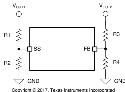
図 6-1. Output Voltage Tracking
