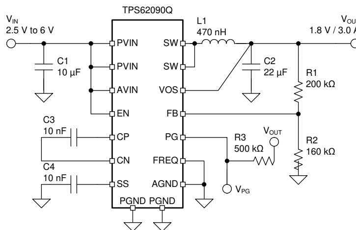
图 7-1. Test Circuit
