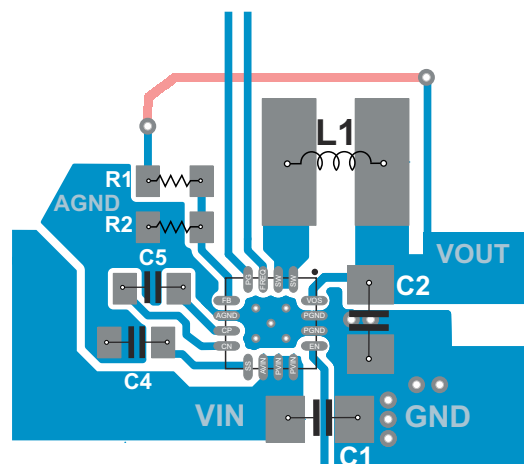
図 7-25. TPS62090Q Layout
