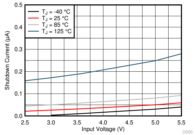
図 6-4. Shutdown Current
