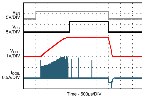
図 8-28. PSM Operation
