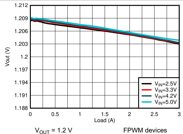
図 8-14. Load Regulation
