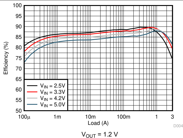
図 8-11. Efficiency
