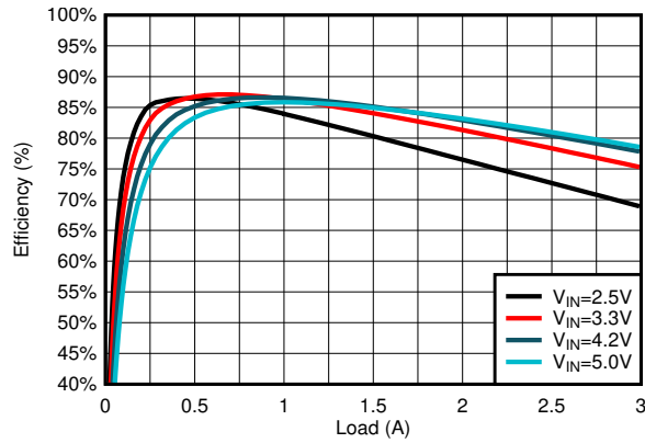
図 8-9. Efficiency
