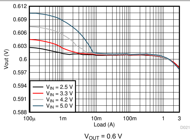
図 8-4. Load Regulation
