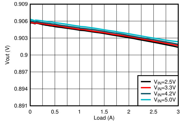
図 8-10. Load Regulation
