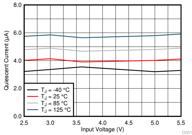
図 6-3. Quiescent Current
