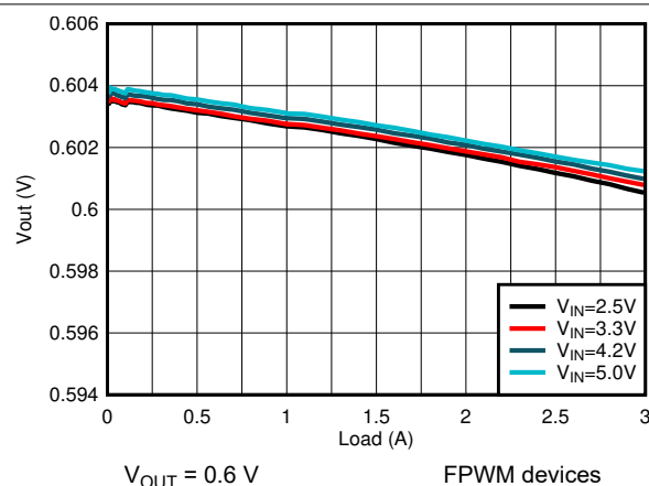
図 8-6. Load Regulation
