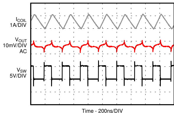
図 8-27. PWM Operation
