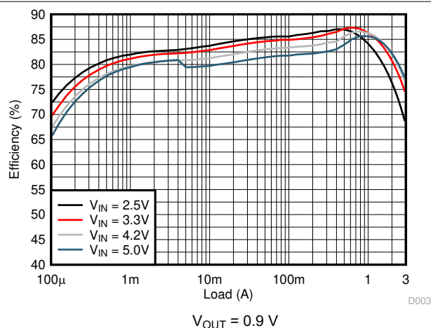
図 8-7. Efficiency
