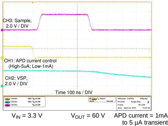
图 13. APD current transient
