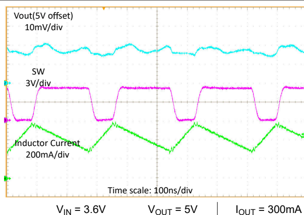
図 8-16. 重負荷時のスイッチング波形
