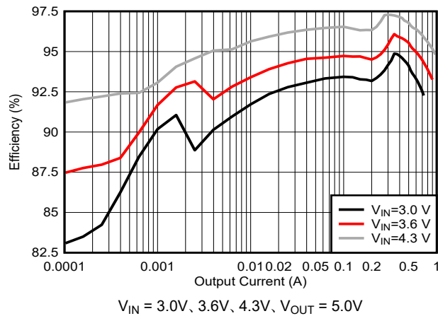
図 6-5. 高速モードにおける異なる入力での 5.0V V_{OUT} の効率
