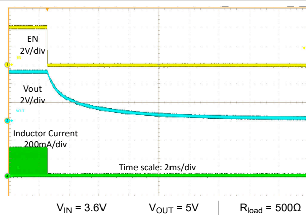
図 8-18. EN によるシャットダウン
