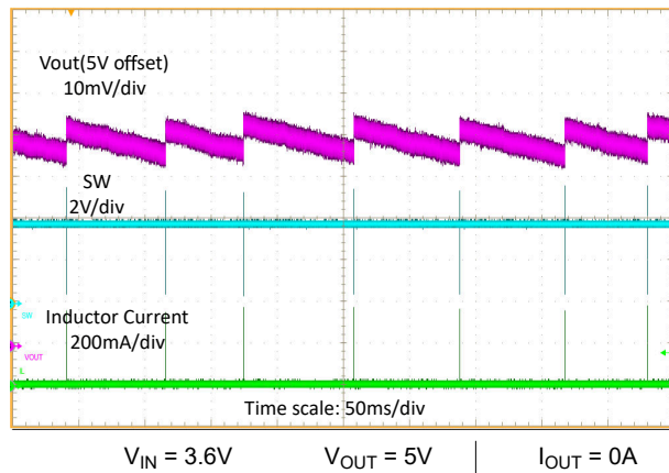
図 8-2. 開放負荷時のスイッチング波形
