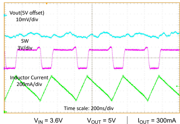
図 8-5. 重負荷時のスイッチング波形
