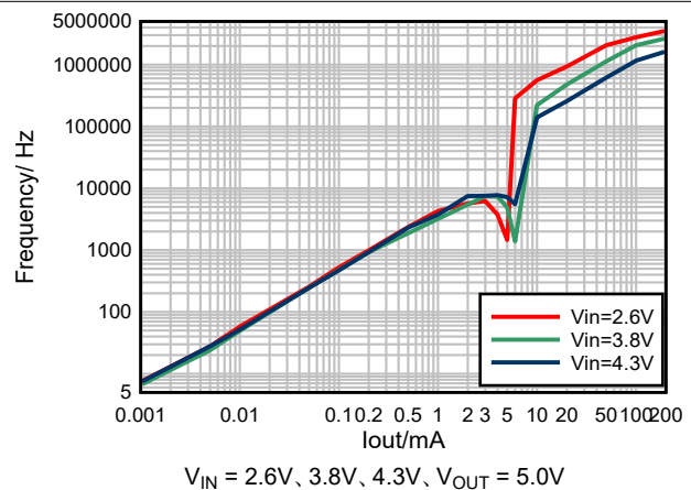
図 6-8. 5.0V V_{OUT} 周波数と通常モードでの出力電流との関係
