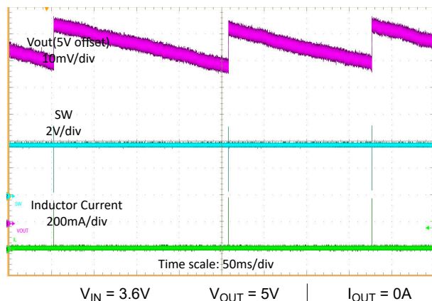
図 8-13. 開放負荷時のスイッチング波形
