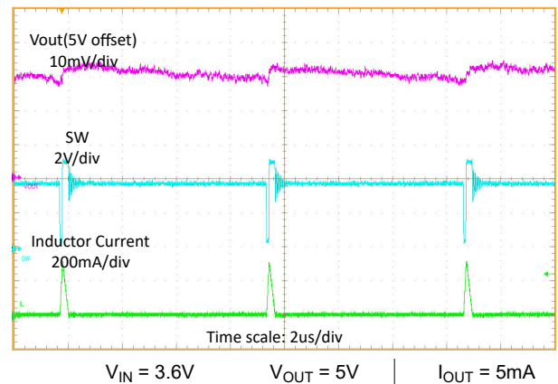
図 8-3. 軽負荷時のスイッチング波形
