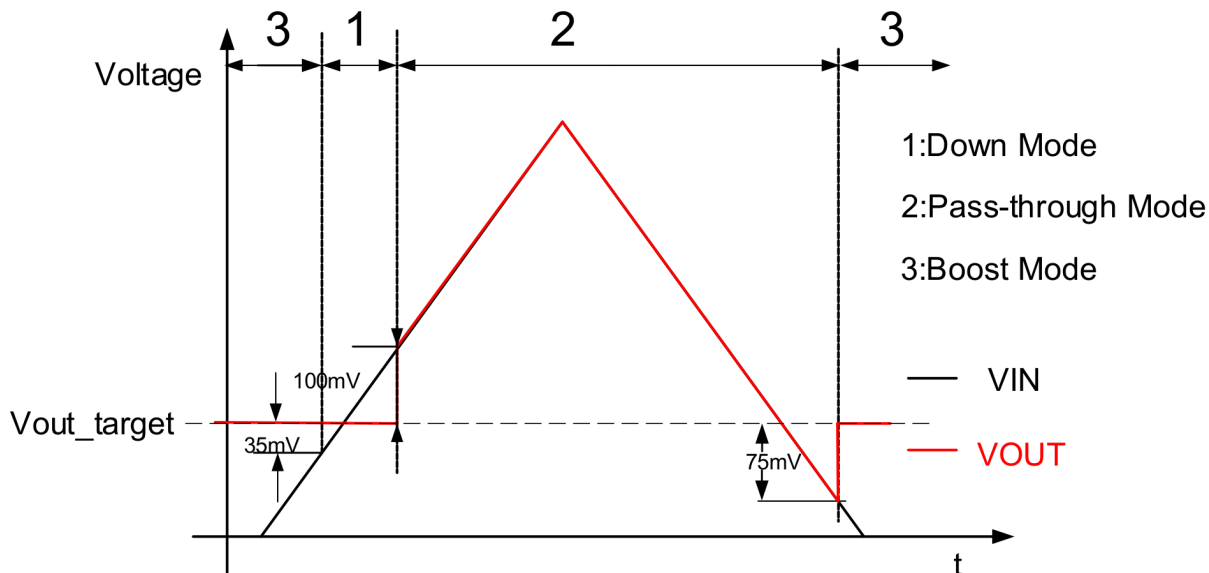
図 7-4. 250mA 以上の入力電流制限バージョンでのモード遷移
