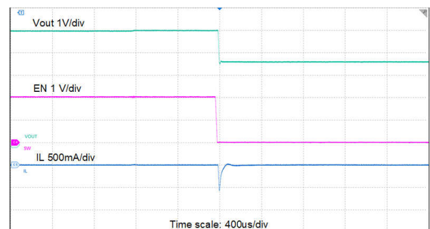
図 8-25. EN によるシャットダウン
