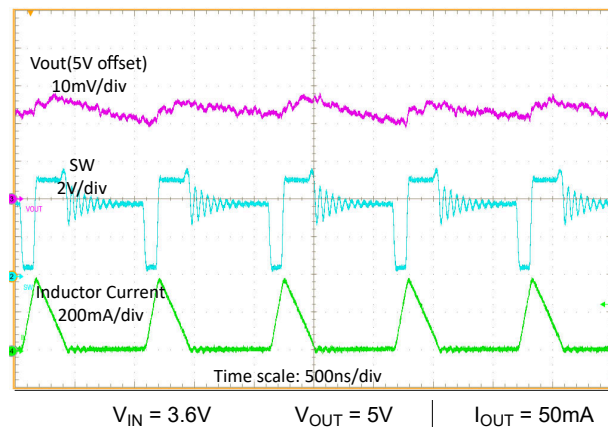
図 8-4. 中負荷時のスイッチング波形
