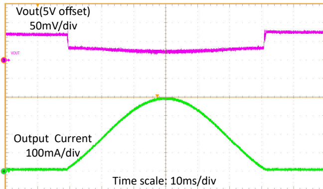
図 8-20. 負荷スweep
