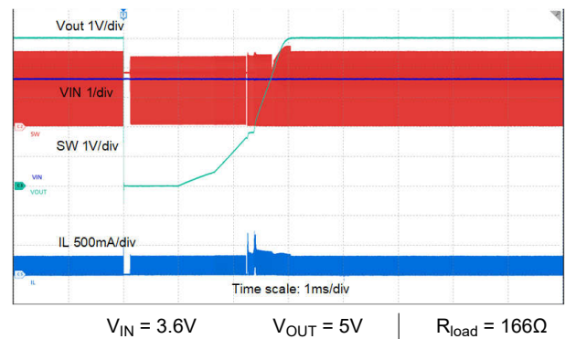
図 8-27. 短絡からの回復
