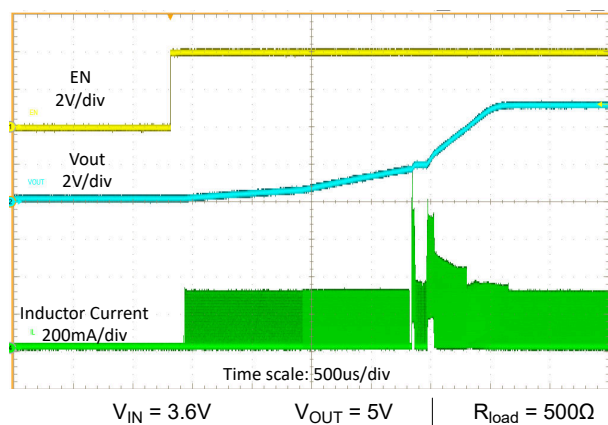
図 8-6. EN によるスタートアップ
