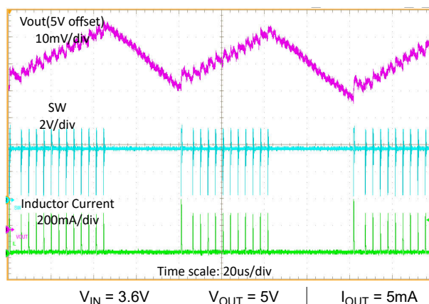
図 8-14. 軽負荷時のスイッチング波形
