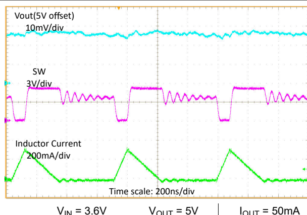
図 8-15. 中負荷時のスイッチング波形
