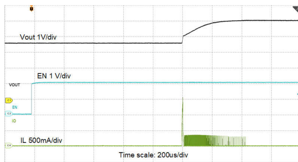
図 8-24. EN によるスタートアップ
