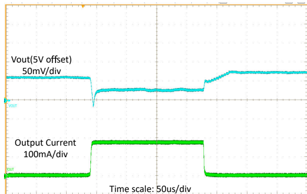
図 8-19. 負荷過渡
