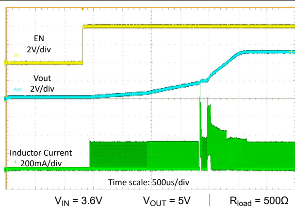
図 8-17. EN によるスタートアップ
