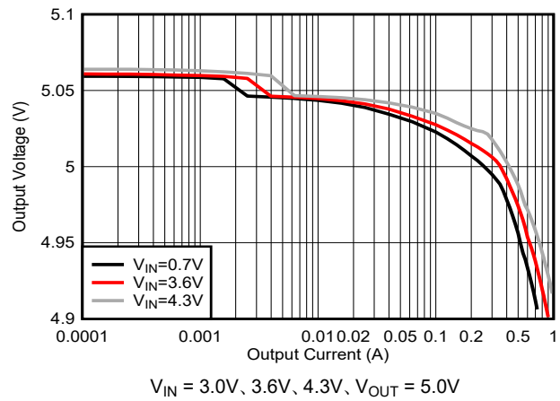
図 6-6. 高速モードにおける異なる入力での 5.0V V_{OUT} のロードレギュレーション
