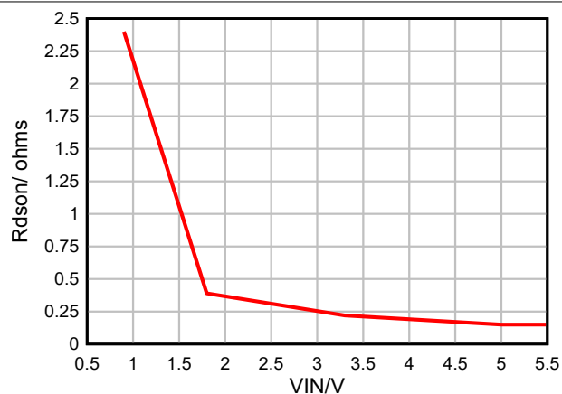
図 6-10. TPS61299A ハイサイド R_{dson} と V_{in} との関係
