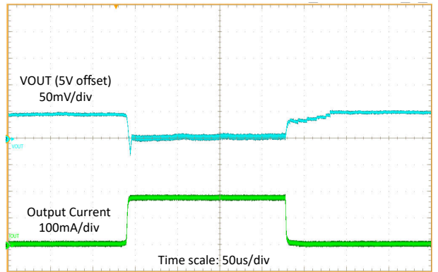
図 8-8. 負荷過渡
