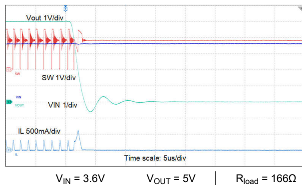
図 8-26. 短絡保護
