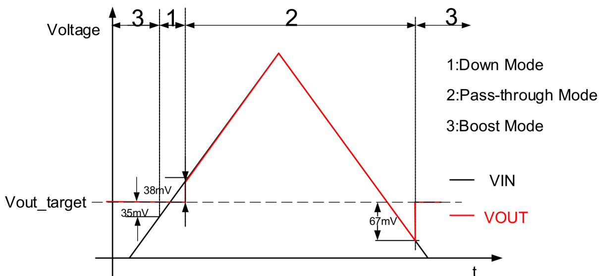
図 7-5. 100mA 以下の入力電流制限バージョンでのモード遷移
