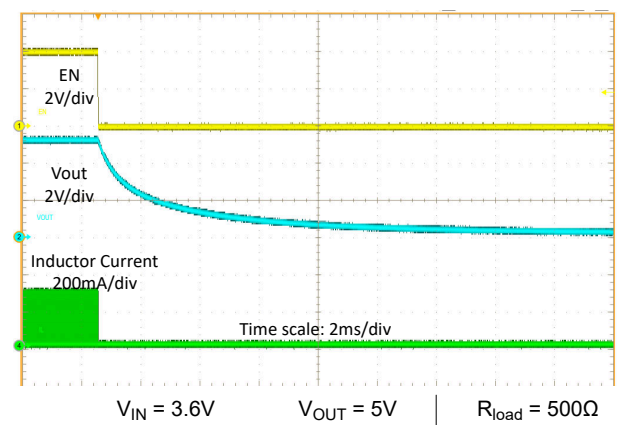
図 8-7. EN によるシャットダウン
