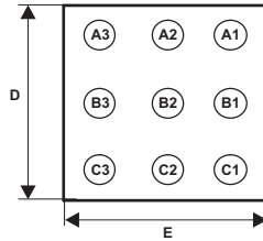
チップ・スケール・パッケージ (底面図)
