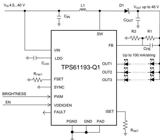
概略回路図
