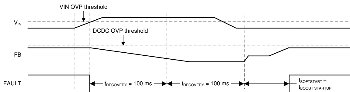
FIG 7-6. V_{IN} Overvoltage Protection ( V_{IN} OVP)
