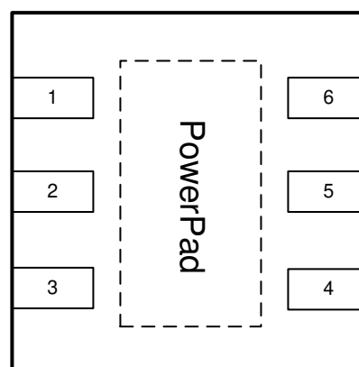
图 6-2. DRV Package 6-Pin DRV Top View
