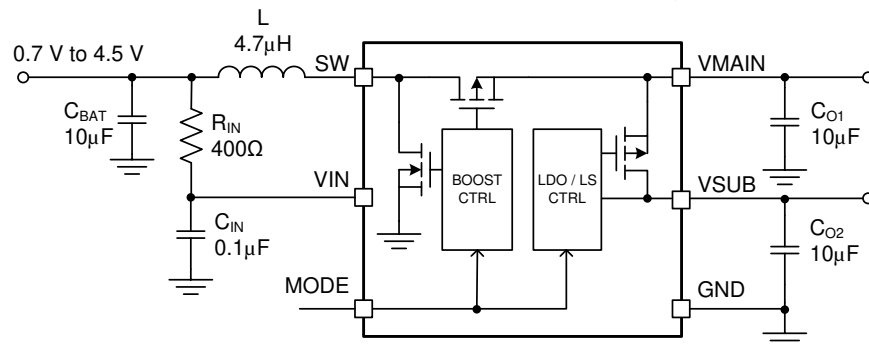
概略回路図
