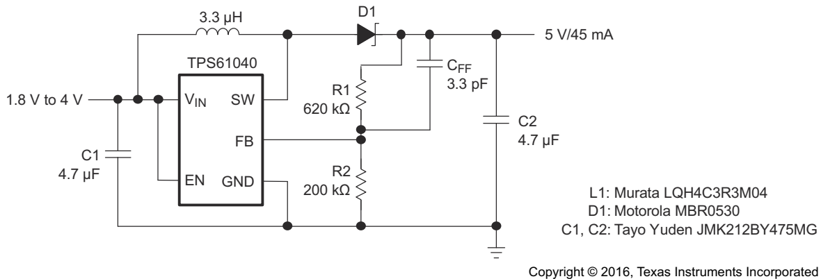
図 8-9. デュアル・バッテリー・セルから 5V/50mA への変換効率は V_{IN} = 2.4V から V_O = 5V/45mA で 約 84%
