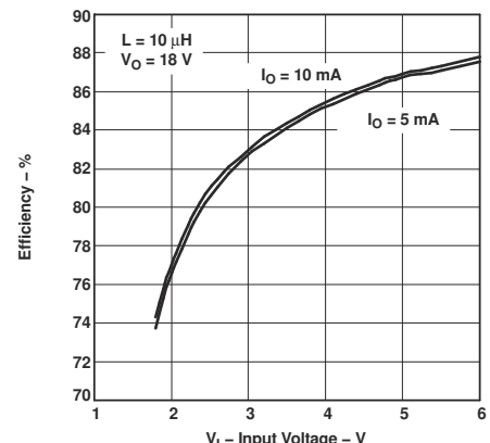
図 6-4. 効率と入力電圧との関係
