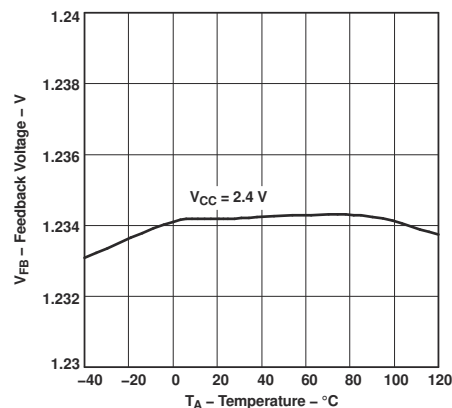
図 6-6. 帰還電圧と自由気流温度との関係
