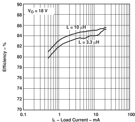
図 6-3. 効率と負荷電流との関係
