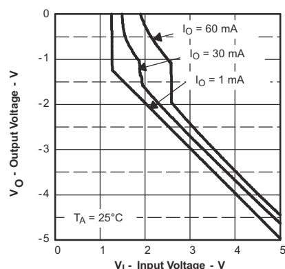
出力電圧と入力電圧との関係
