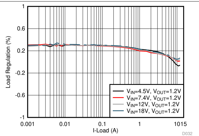
図 20. Load Regulation
