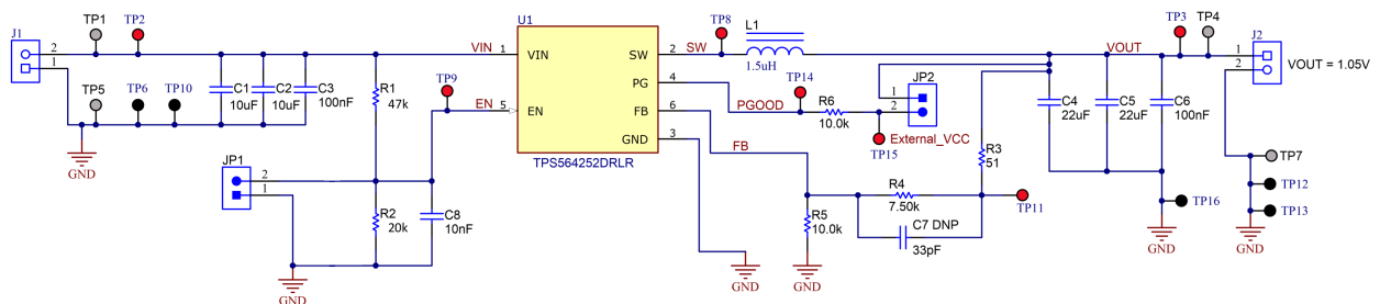
図 8-1. Schematic
