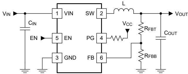
簡素化されたアプリケーション
