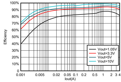
TPS564252 の効率 ( V_{IN} = 12V )
