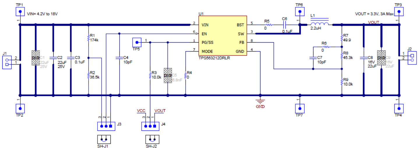
図 8-1. TPS563212 3.3-V, 3-A Reference Design
