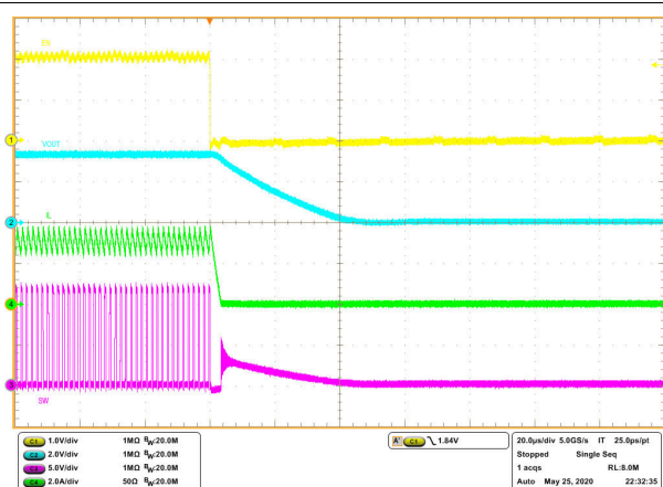
图 8-19. Disable Relative to EN
