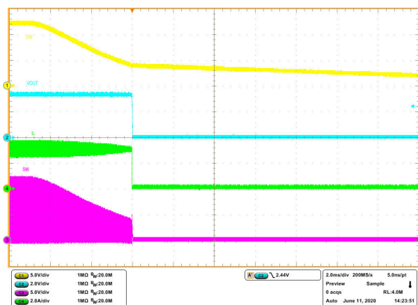
图 8-17. Shutdown Relative to VIN
