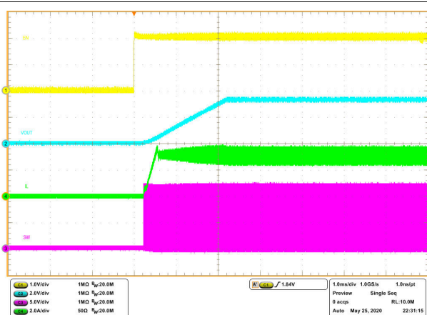
图 8-18. Enable Relative to EN
