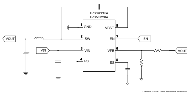
概略回路図
