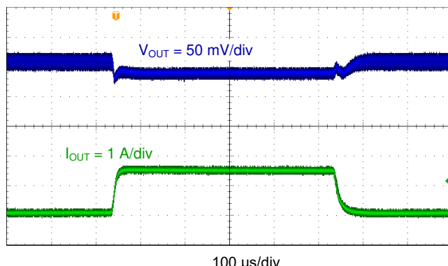
図 7-11. TPS563201 Transient Response, 0.1 to 1.5 A
