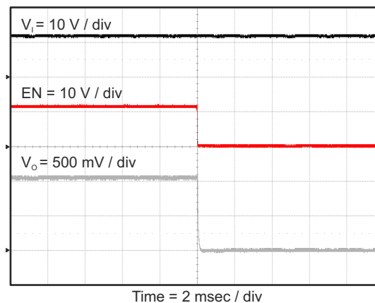
図 8-15. Tps562200 Shut Down Relative to En
