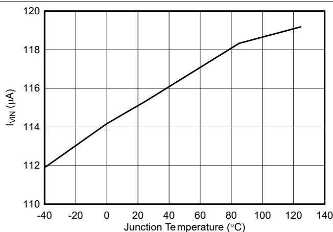
図 5-1. TPS562243 Quiescent Current
