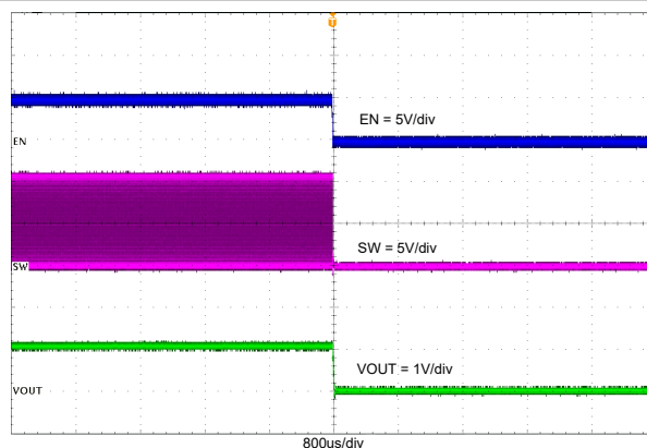
図 7-7. TPS562243 Enable Off With 2A Loading
