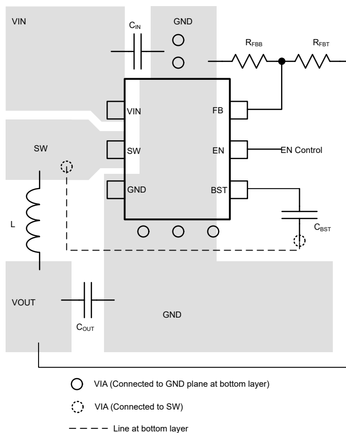
図 7-18. TPS56224x Layout
