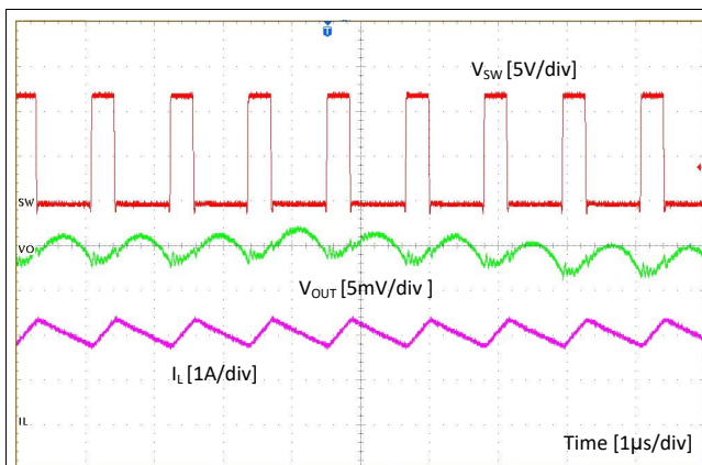
14. CCM Mode
