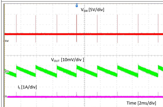
16. PSM Mode
