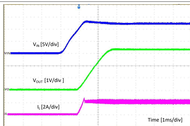
15. DCM Mode
