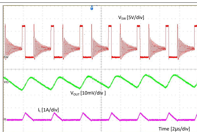
15. DCM Mode
