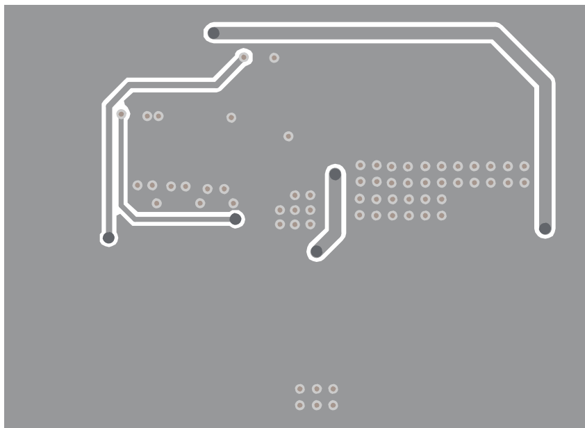
FIG 10-2. Bottom Layout Example
