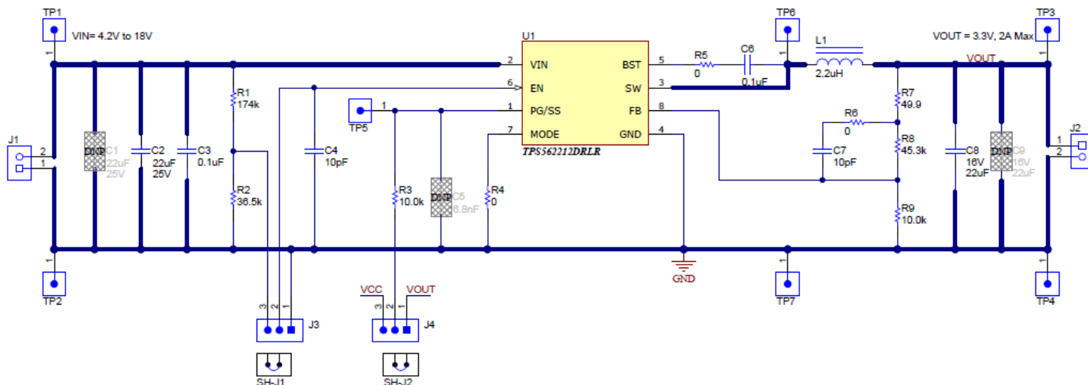
図 8-1. TPS562212 3.3-V, 2-A Reference Design
