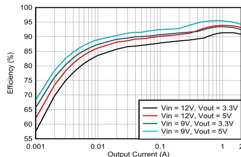
効率と出力電流との関係
