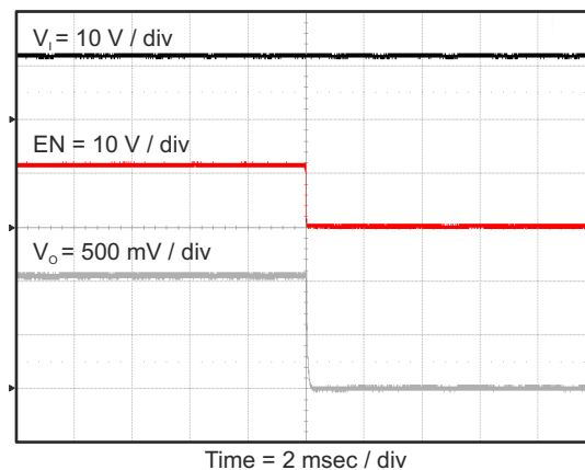
図 8-15. Tps562200 Shut Down Relative to En
