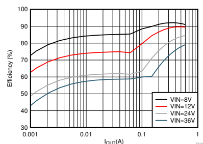
効率と出力電流との関係 V_{OUT} = 5V 、2100kHz、PFM
