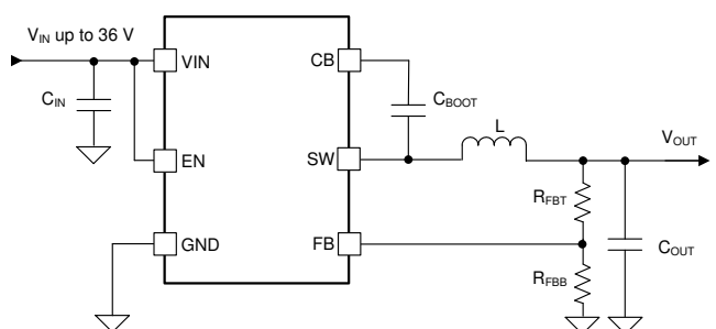
概略回路図
