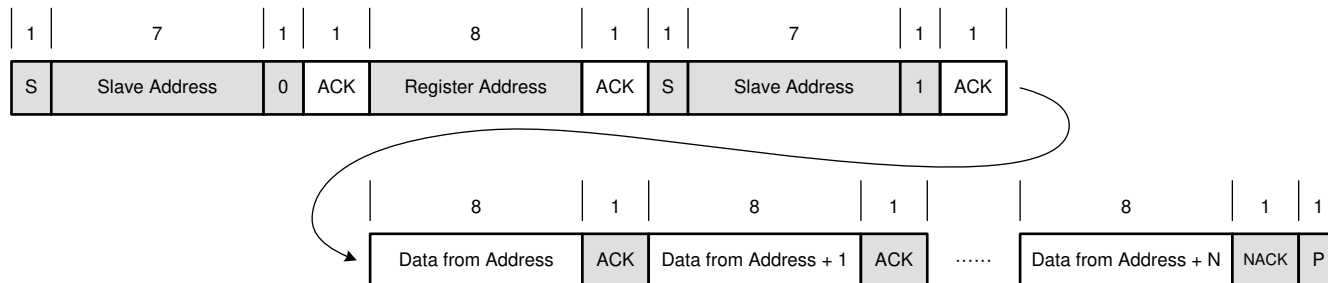
图 7-14. Multi-byte Read
