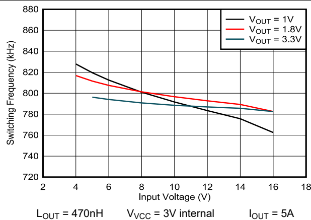
図 5-9. 800kHz Switching Frequency versus Input Voltage
