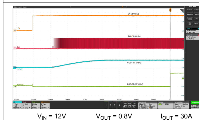
図 7-10. Start-Up With EN
