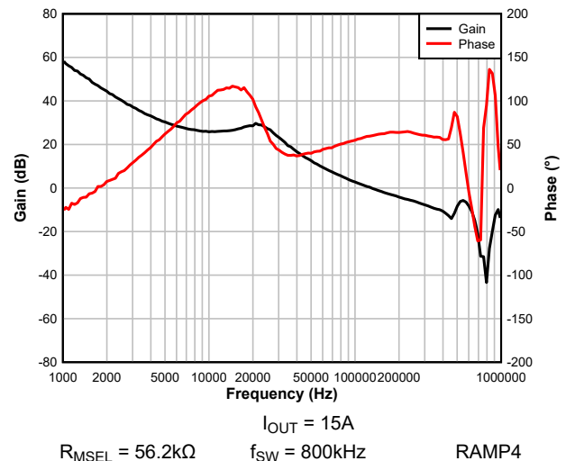
図 7-7. Bode Plot
