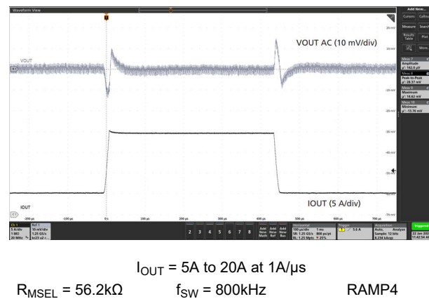
図 7-6. Load Transient
