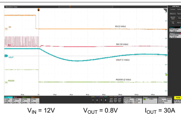
図 7-11. Shutdown With EN
