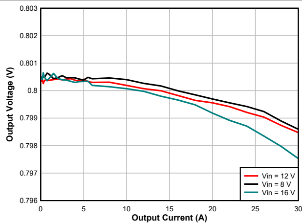
図 7-4. Load Regulation
