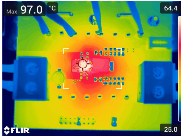
図 5-7. Thermal Image – 0.8V Output, TPS54KC23EVM, 6 Layers
