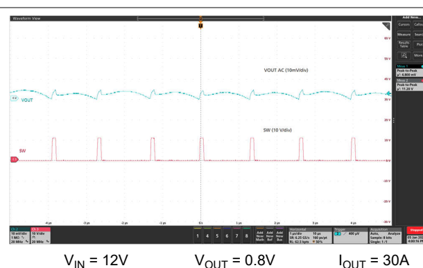
図 7-9. Output Voltage Ripple – FCCM
