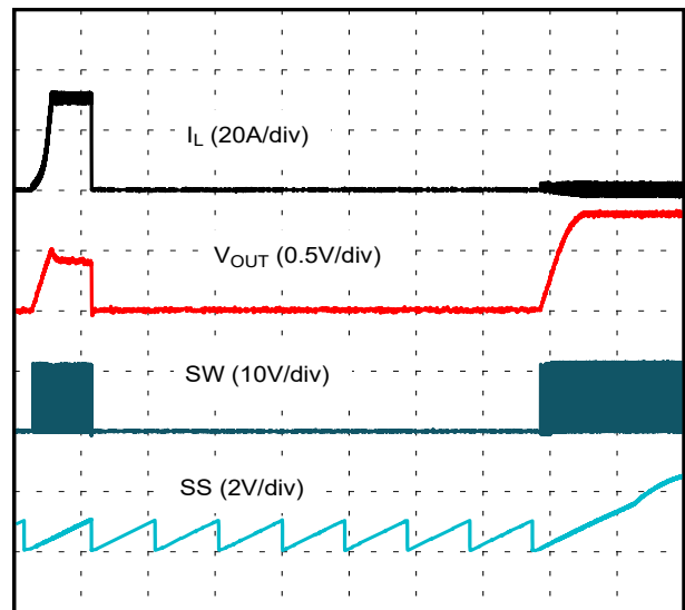
図 6-2. Exiting Hiccup
