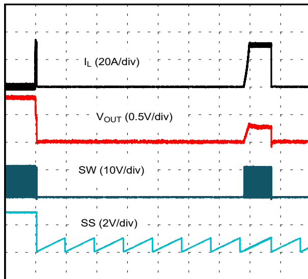
図 6-1. Entering Hiccup
