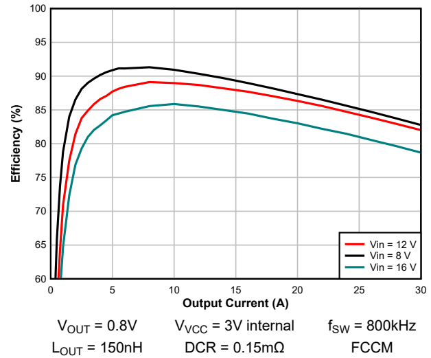
図 7-3. Efficiency – FCCM
