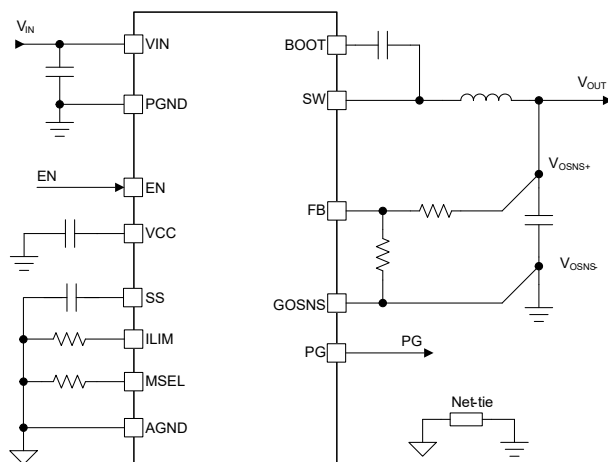
概略回路図
