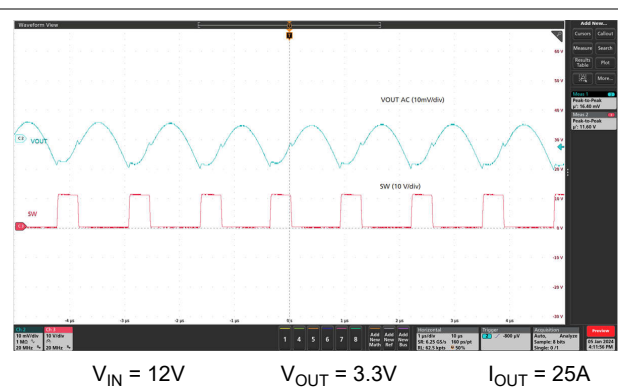
図 7-9. Output Voltage Ripple – FCCM
