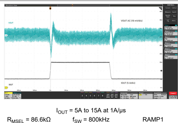
図 7-6. Load Transient
