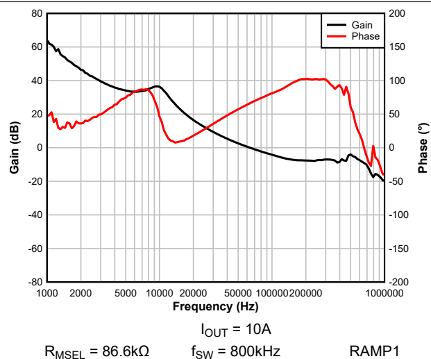
図 7-7. Bode Plot
