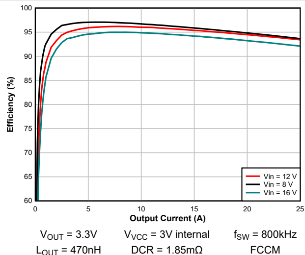
図 7-3. Efficiency – FCCM
