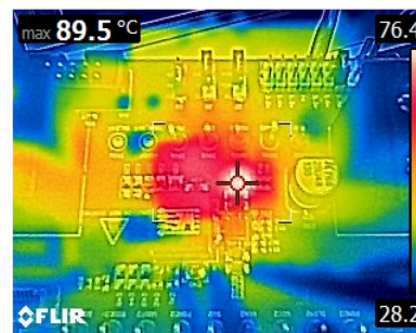
図 5-8. Thermal Image – 3.3V Output, TPS54KB20EVM, 6 Layers
