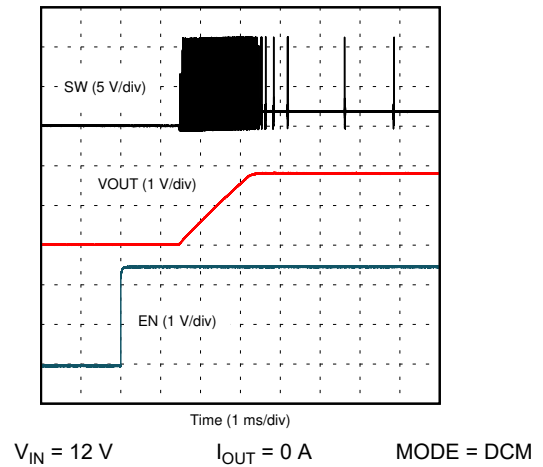
図 7-17. EN Start-Up – DCM
