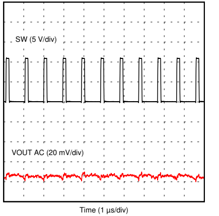
図 7-26. Output Voltage Ripple
