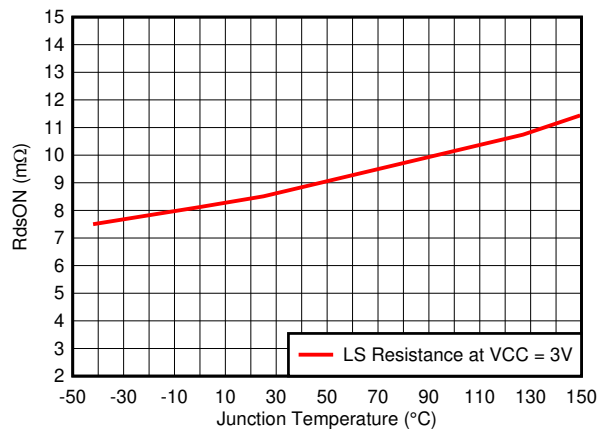
図 5-2. Low-Side FET RdsON
