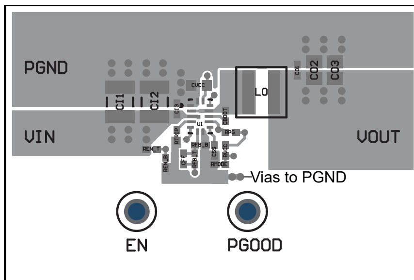
図 7-31. Top Layer Layout
