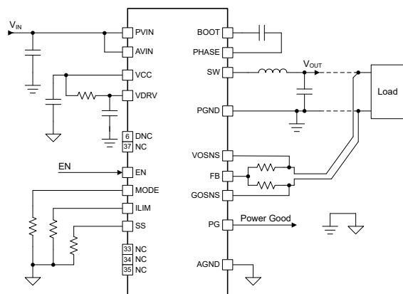
概略回路図
