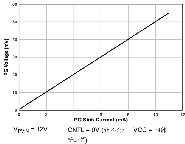
図 5-3. PGOOD の I-V 曲線
