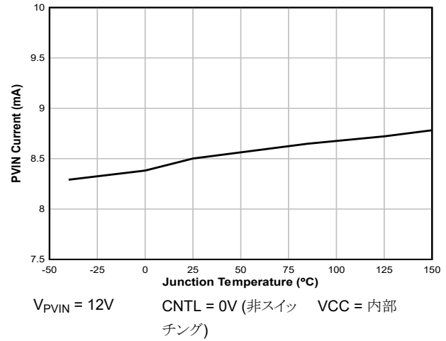
図 5-2. VIN Iq と接合部温度との関係
