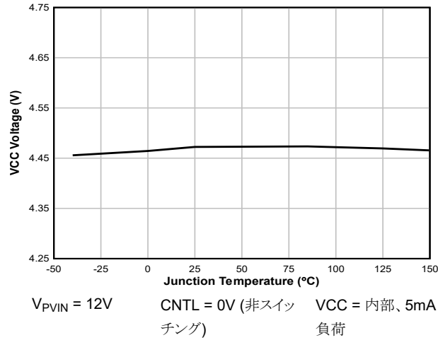
図 5-1. VCC LDO と接合部温度との関係
