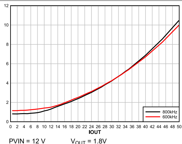
図 8-11. 消費電力、FFCM、外部 5V バイアス
