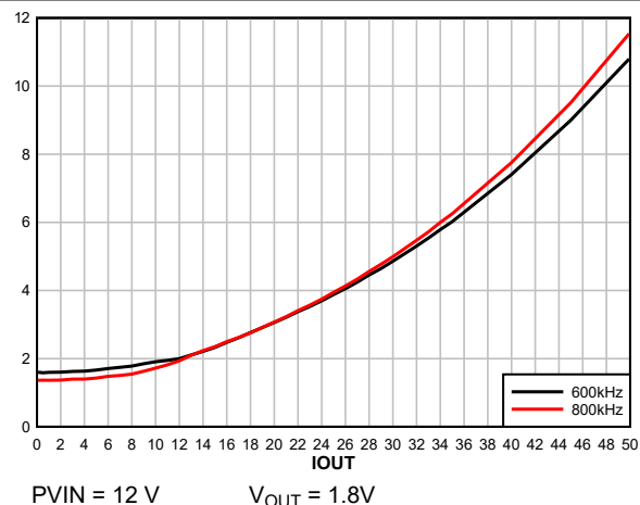
図 8-9. 消費電力、FFCM、内部 LDO
