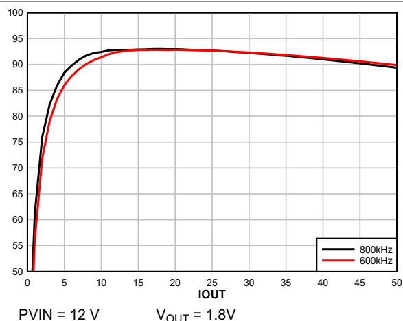
図 8-10. 効率、FFCM、外部 5V バイアス
