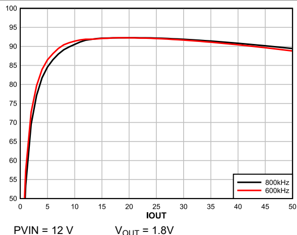
図 8-8. 効率、FFCM、内部 LDO
