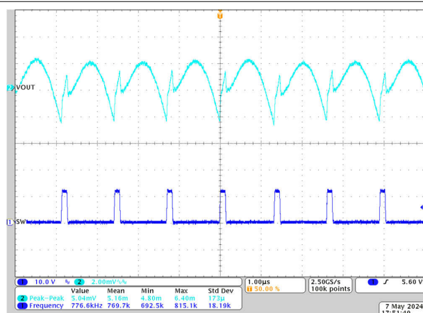
図 8-16. 出力電圧リップル、1.2V Vout、800kHz FCCM、25A 負荷
