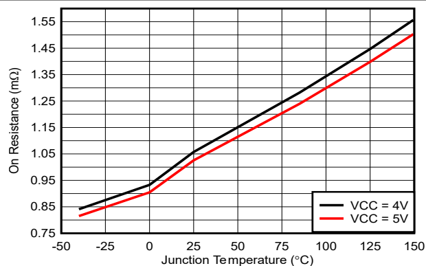
図 5-4. ローサイド MOSFET オン抵抗 ( R_{DS(on)} ) と接合部温度との関係
