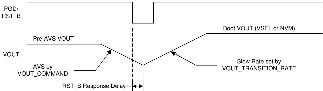
FIG 7-7. TPS546D24S Output Voltage Reset
