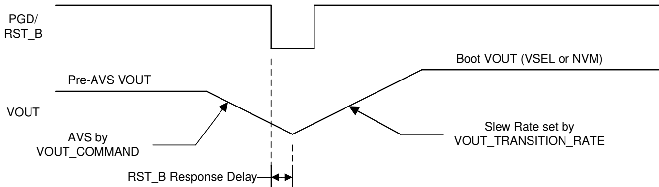
FIG 7-7. TPS546D24A Output Voltage Reset
