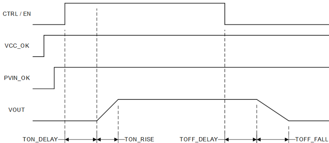
図 6-4. TPS546B25 のスタートアップとシャットダウン
