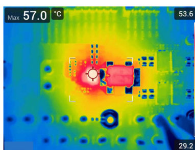
図 8-7. 熱特性、800kHz FCCM、外部 5V バイアス、25A 負荷
