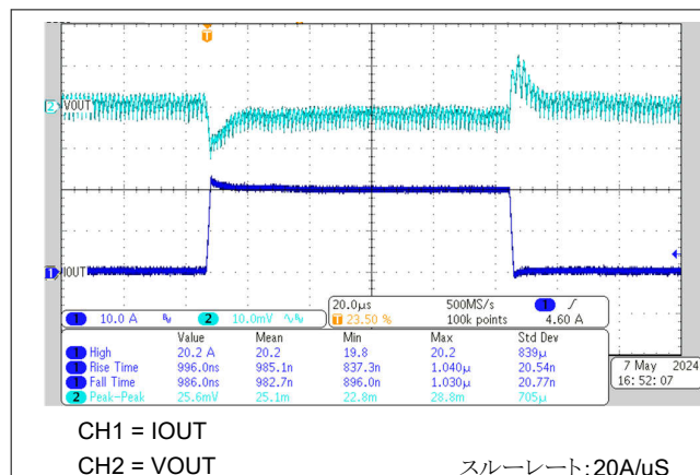
図 8-2. 負荷過渡応答 0A ~ 20A
