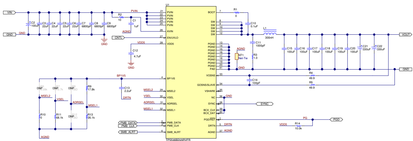
図 8-1. TPS546B24A Application
