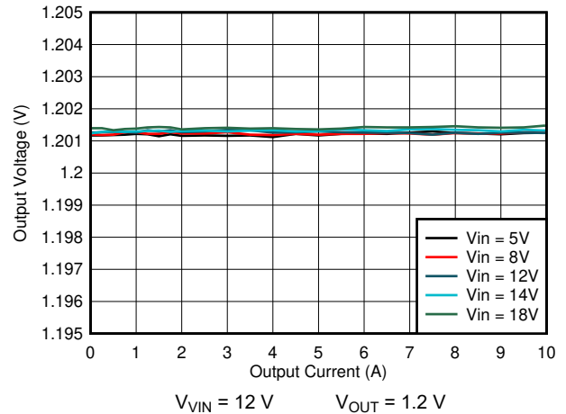
図 7-3. Load Regulation
