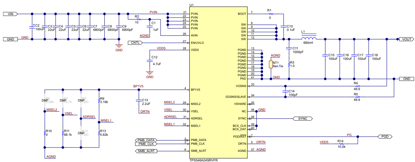
図 7-1. TPS546A24S Application
