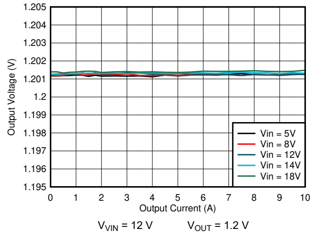
图 8-3. Load Regulation
