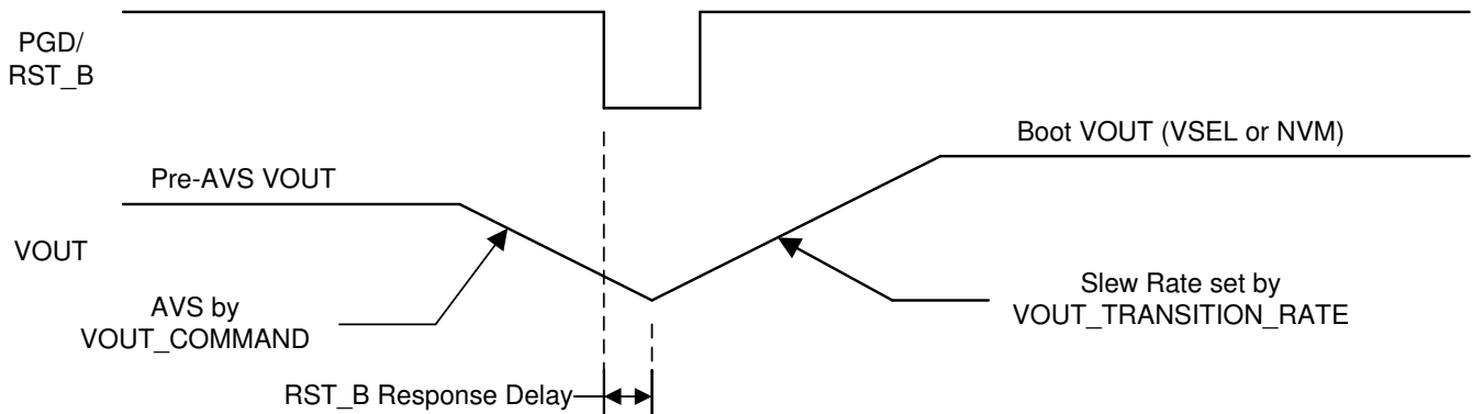
图 7-7. TPS546A24A Output Voltage Reset
