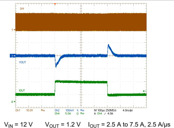
图 8-7. Load Transient Response
