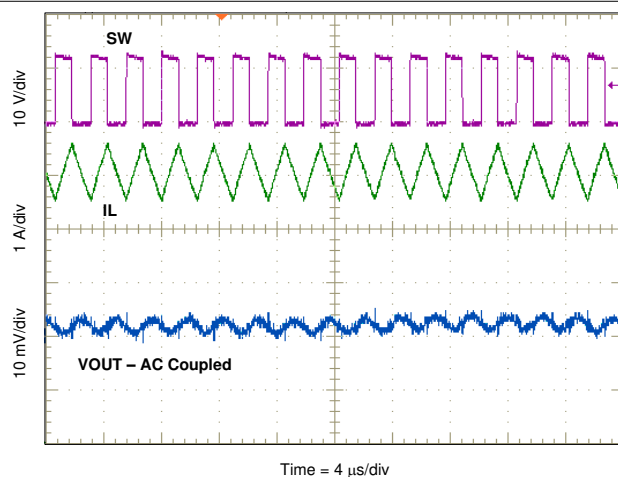
8-10. Output Ripple CCM
