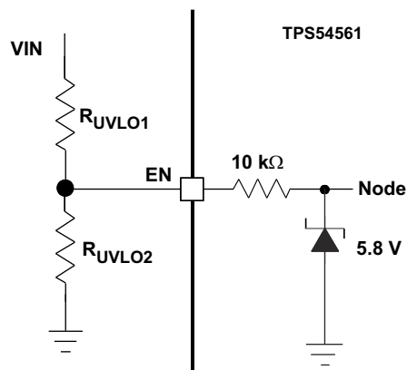
7-2. Internal EN Pin Clamp
