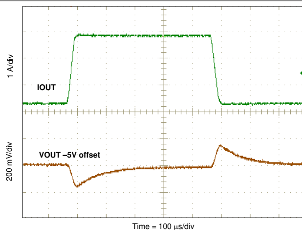
8-6. Load Transient
