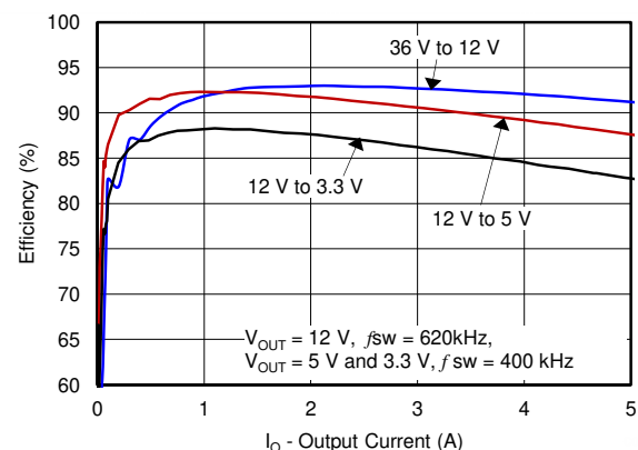
効率と負荷電流との関係
