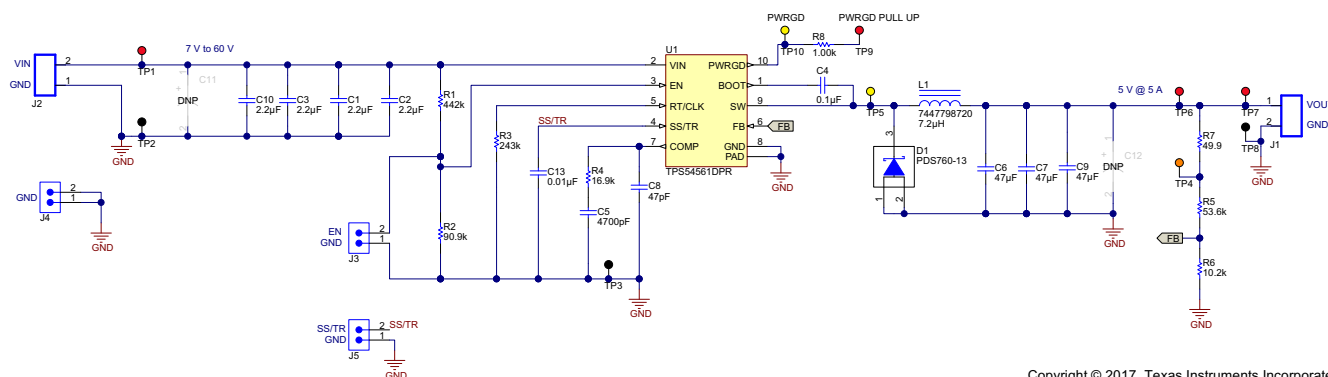
图 8-1. 5-V Output TPS54561 Design Example
