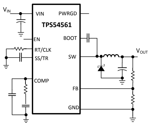
概略回路図
