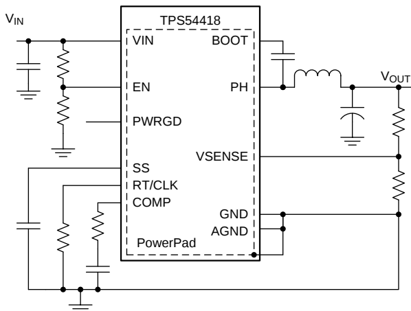
概略回路図
