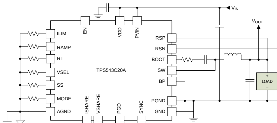
概略回路図
